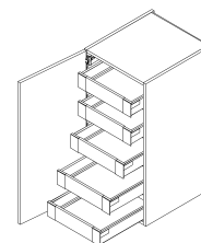
Art.Bez.: TLI5 Korpus mit Tür und 5 Innenladen (mit Aufopplung 25 mm)
