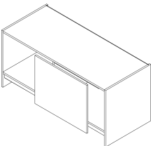
Art.Bez.: S37 Korpus mit Schiebetür rechts (UL) offen links mit Beschlag Frontino 20 H (max. 20kg Türgewicht)
