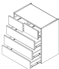
Art. Bez.: L15 Korpus mit 3 Lade und 1 Doppellade, mit Mittelboden und Mittelseite, Doppellade ist mittig geteilt
