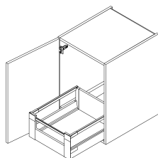
Art.Bez.: TLI1 Korpus mit Tür und 1 Innenlade (mit Aufopplung 25 mm)
