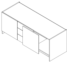
Art.Bez.: S27 Korpus mit Schiebetüren (UL) 3 Laden mittig
