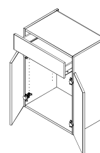
Art.Bez.: TL12 Korpus mit 1 Doppeltür und 1 Lade, mit Mittelboden
