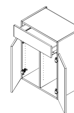
Art.Bez.: TL13 Korpus mit 1 Doppeltür und 1 Lade, mit Mittelboden und Mittelseite
