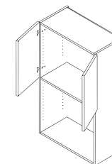
Art.Bez.: T13 Korpus mit Mittelboden, Doppeltür, unten offen
