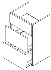
Art. Bez.: G20 Korpus für Kochfeld mit 2 Laden und Frontblende
