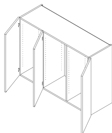
Art.Bez.: T15 Korpus mit 3 Türen und 2 Mittelseiten
