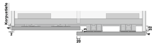
Detail 2 zu S11 (S12 Ansicht gespiegelt)
