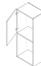
Art.Bez.: T14 Korpus mit Mittelboden, Tür, unten offen
