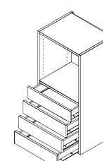
Art. Bez.: L20 Offener Korpus mit 4 Lade, mit Mittelboden
