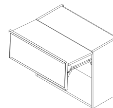
Art.Bez.: T19 Aventos Hochfaltklappe (HF) mit unterschiedlichen Frontausführungen
