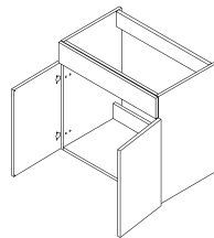
Art.Bez.: G2 Spülenkorpus mit 1 Doppeltür, Frontblende und stehender Traverse
