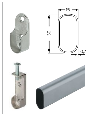
Kleiderstange chromfärbig inkl. 2 Halterungen
