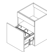
Art. Bez.: G38 Spülenkorpus mit Müllauszug Cargo grau, Frontblende und stehender Traverse
