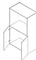
Art.Bez.: T11 Korpus mit Mittelboden, Doppeltür, oben offen
