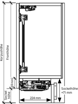
Detail zu S25 bis S37
