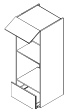
Art.Bez.: G13 Korpus mit 1 Lade, E-Herd, Mikrowelle und 1 Klappe, mit 3 Mittelböden
