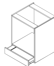
Art.Bez.: G3 Korpus mit 1 Lade und E-Herd, mit Mittelboden und oben Traverse
