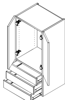
Art.Bez.: TL10 Korpus mit 3 Läden und 1 Doppel- tür, mit Mittelboden
