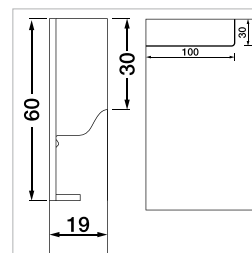
Detail zu PVGM und PVGM Alu-Niro geb.
