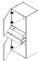
Art.Bez.: TL16 Korpus mit 2 Türen und 2 Läden mittig, mit 2 Mittelböden
