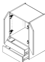
Art.Bez.: TL9 Korpus mit 2 Läden und 1 Doppel- tür, mit Mittelboden
