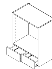
Art. Bez.: L21 Offener Korpus mit 1 Doppellade, mit Mittelboden und Mittelseite, Doppellade ist mittig geteilt
