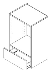
Art. Bez.: L17 Offener Korpus mit 1 Lade, mit Mittelboden
