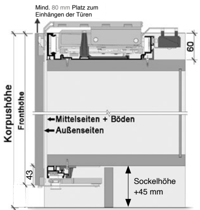
Detail zu S40 bis S43
