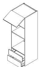
Art.Bez.: G14 Korpus mit 2 Läden, E-Herd, Mikrowelle und 1 Klappe, mit 3 Mittelböden
