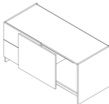
Art.Bez.: S34 Korpus mit Schiebetür rechts (UL) und 2 Laden links
