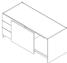
Art.Bez.: S35 Korpus mit Schiebetür rechts (UL) und 3 Laden links
