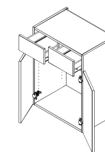
Art.Bez.: TL14 Korpus mit 1 Doppeltür und 1 Doppel- lade, mit Mittelboden und Mittelseite, Doppellade ist mittig geteilt
