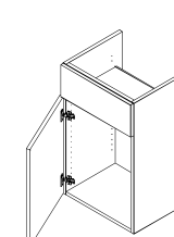
Art.Bez.: G19 Korpus für Kochfeld mit 1 Tür und 1 Frontblende, mit Mittelboden und stehendem Traver vorne
