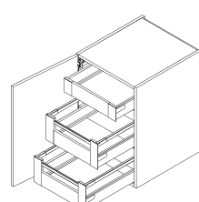
Art.Bez.: TLI3 Korpus mit Tür und 3 Innenladen (mit Aufopplung 25 mm)
