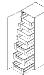
Art.Bez.: TLI7 Korpus mit Tür und 7 Innenladen (mit Aufopplung 25 mm)
