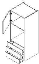
Art.Bez.: G6 Korpus mit 3 Läden, E-Herd und 1 Tür, mit 2 Mittelböden
