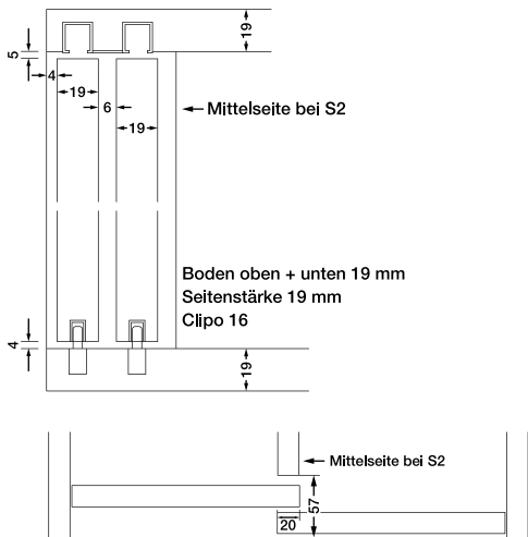
Detail zu S1 und S2
