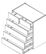
Art. Bez.: L16 Korpus mit 4 Lade und 1 Doppellade, mit Mittelboden und Mittelseite, Doppellade ist mittig geteilt
