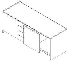
Art.Bez.: S28 Korpus mit Schiebetüren (UL) 4 Laden mittig
