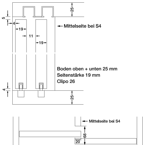
Detail zu S3 und S4
