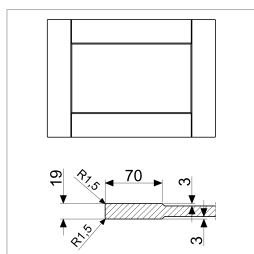
Modell PVR70 Rahmentür mit 70 mm Friesbreite
