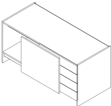
Art.Bez.: S32 Korpus mit Schiebetür links (UL) und 4 Laden rechts
