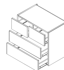
Art. Bez.: L14 Korpus mit 2 Lade und 1 Doppellade, mit Mittelboden und Mittelseite, Doppellade ist mittig geteilt
