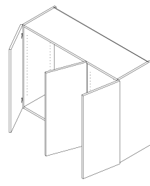
Art.Bez.: T17 Korpus mit Doppeltür links, 1 Tür rechts und 1 Mittelseite
