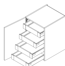
Art.Bez.: TLI4 Korpus mit Tür und 4 Innenladen (mit Aufopplung 25 mm)
