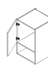
Art.Bez.: G18 Korpus für Mikrowelle mit 1 Tür, mit Mittelboden
