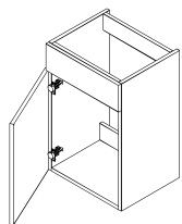
Art.Bez.: G1 Spülenkorpus mit 1 Tür, Frontblende und stehender Traverse
