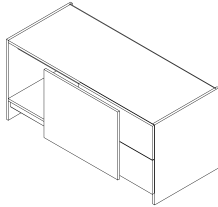
Art.Bez.: S30 Korpus mit Schiebetür links (UL) und 2 Laden rechts
