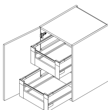
Art.Bez.: TLI2 Korpus mit Tür und 2 Innenladen (mit Aufopplung 25 mm)
