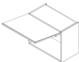
Art. Bez.: T23 Aventos kleine Hochklappe (HK-S)
