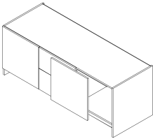
Art.Bez.: S26 Korpus mit Schiebetüren (UL) 2 Laden mittig
