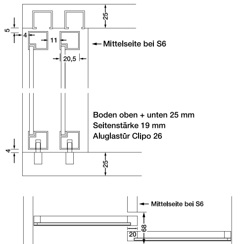
Detail zu S5 und S6
