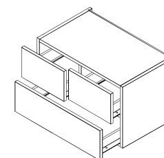
Art. Bez.: L13 Korpus mit 1 Lade und 1 Doppellade, mit Mittelboden und Mittelseite, Doppellade ist mittig geteilt
