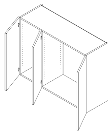
Art.Bez.: T16 Korpus mit Doppeltür rechts, 1 Tür links und 1 Mittelseite
