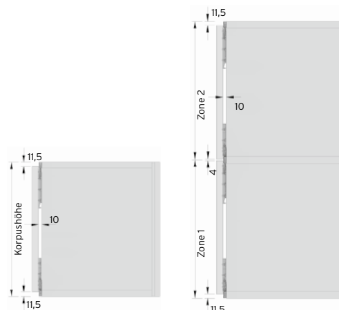
Detail 4 zu S14 und S16
