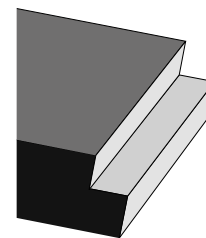
FALZAUSFRÄSUNG/TYP M Bild 32
